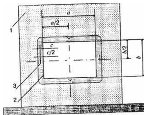
Рисунок А. 2 -Схема размещения вертикальных воздуховодов на испытательном стенде
